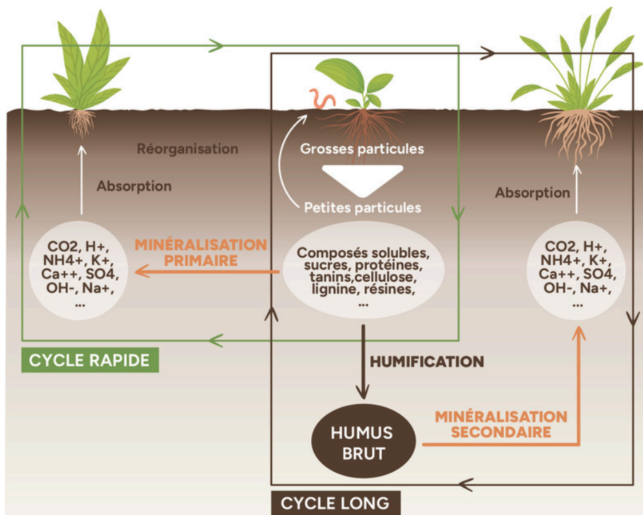
Cycle simplifié de la matière organique dans le sol
